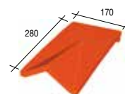
611 V17 Driehoekige ventilatiepan (doorsnede 35 cm 2 )
