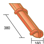
881 XL Stijlvolle eindnoordboom (klein model) - 2,2 kg
