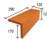
201 P17 Links rechter gevelpan - 2 kg
