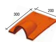
61 P20 Halfronde ventilatiepan (doorsnede 35 cm 2 ) - 1,4 kg
