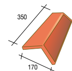
432 EL Hoekige noordboom (hoekkeper) - 1,1 kg
