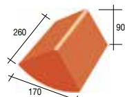
454 XTP Eindnoordboom (of hoekboom) - 1,6 kg
