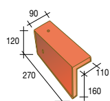
201 EM Linker gevelpan - 6 per lm - 1,9 kg
