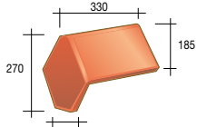
362 XLP Hoekige beginvorst - 3,7 kg
