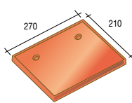
83 EL Gootpan en ondervorstpan - 1,4 kg
