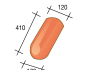
453 XLP Tapse eindnoordboom (klein model) - 1,8 kg
