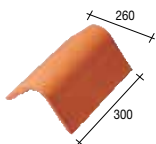
33 XTP Hoekige vorst (doorsnede 25 cm 2 ) - 3,4 per lm - 3 kg
