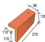
202 PG Rechter gevelpan - 2 kg
