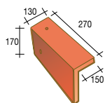
201 EL Linker gevelpan - 3,6 per lm - 2,8 kg
