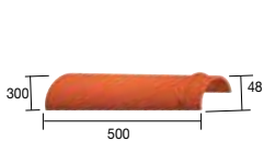
28 XG Sluitvorst 500 mm - 2,2 per lm - 4,3 kg
