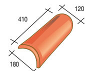
434 XLP Tapse noordboom (klein model) - 1,9 kg
