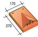
612 NO Driehoekige ventilatiepan met rooster (doorsnede 20 cm 2 ) - 1,2 kg
