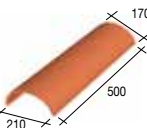
1 CL Kanaalpan Languedocienne - 2,5 per lm - 2,6 kg
