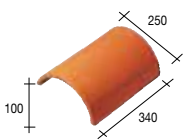
34 XTP Halfronde vorst "Val de Loire" - 3 per lm - 3,3 kg
