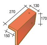
202 EL Rechter gevelpan - 3,6 per lm - 2,8 kg
