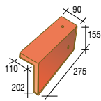
202 XLP Rechter gevelpan - 6 per lm - 1,8 kg
