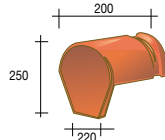
366 XL Halfronde ventilerende eindschubvorst - 3,4 kg
