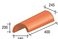
336 XL Beginvorst / noordboom met schacht (groot model) - 3,2 kg
