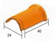
31 XL Halfronde ventilerende sluitvorst 2,5 per lm - 4,1 kg
