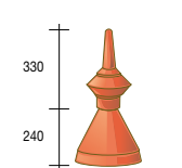
483 XL Sierstuk spits - 2,3 kg 482 XL Voet sierstuk spits - 3,9 kg
