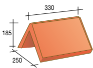
33 XLP Hoekige vorst - 3 per lm - 3,1 kg
