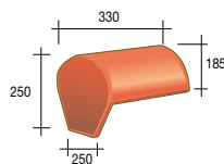
365 XLP Halfronde beginvorst - 4,1 kg
