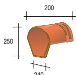
366 XL Halfronde ventilerende eindshubvorst - 3,4 kg
