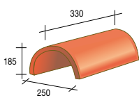
34 XLP Halfronde vorst - 3 per lm - 3,1 kg
