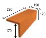
201 V17 Links rechter gevelpan - 5 per lm - 2 kg
