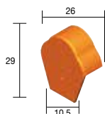
367 XT Begin-en eindvorst Résidence - 2,4 kg
