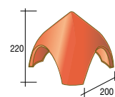
462 XL Kap 1 vorst / 2 noordbomen - 3,4 kg
