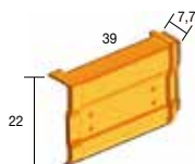
203 XL Universele gevelpan - 2,6 per lm - 3,6 kg
