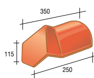
472 XLP Kap 1 halfronde vorst - 2 noordbomen - 4,5 kg
