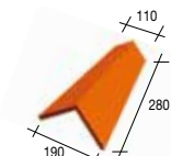
432 XGP Hoekige noordboom (nieuw model) - 1,6 kg
