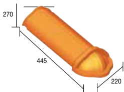
Eindnoordboom Résidence - 2,4 kg
