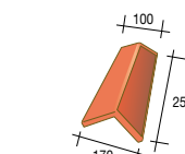
43 EM Ingecapselde hoekige noordboom - 11 per lm - 1 kg
