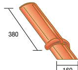
327 XL Stijlvolle eindnoordboom met sluiting (klein model) - 2,6 per lm - 2,9 kg
