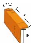
16 XLD Linker gevelpan - 3,8 kg - 2,5 per lm
