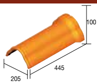
321 XT Ronde vorst Résidence + klem - 2,5 per lm - 3,6 kg
