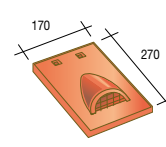
613 EM Ventilatiepan met rooster (doorsnede 35 cm 2 ) - 1,7 kg
