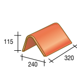
33 XLP Hoekige vorst - 3 per lm - 3,1 kg
