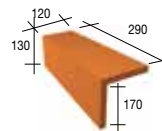
201 BG Linker gevelpan
