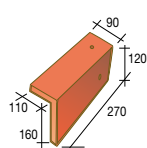
202 EM Rechter gevelpan - 6 per lm - 1,9 kg
