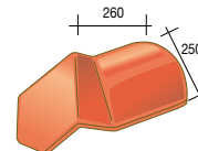
472 XLP Kap 1 halfronde vorst 2 noordbomen - 4,5 kg
