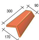
433 XTP Gevelpan (of hoekpan) - 1,6 kg
