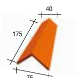
433 XL Ingewerkte hoekige noordboom - 11 per lm - 1,10 kg
