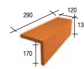
202 BG Rechter gevelpan
