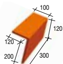
201 P20 Links rechter gevelpan - 2,4 kg
