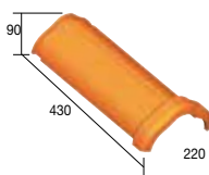
32 XT Noordboom Résidence - 3 per lm - 2,85 kg
