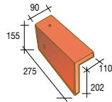
201 XLP Linker gevelpan - 6 per lm - 1,8 kg
