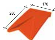
611 P17 Driehoekige ventilatiepan (doorsnede 35 cm 2 ) - 1,5 kg
