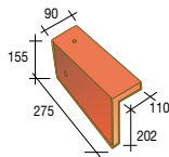
201 NO Linker gevelpan - 6 per lm - 1,6 kg
