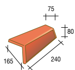
432 XL Hoekige noordboom - 11 per lm - 1,1 kg
