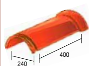
31 XL Halfronde ventilerende sluitvorst - 2,5 per lm - 4,1 kg
