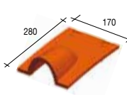
61 P17 Halfronde ventilatiepan (doorsnede 35 cm 2 ) - 1,5 kg
