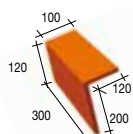
202 P20 Links linker gevelpan - 2,4 kg
