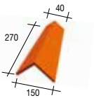
433 NO Noordboom met sluiting - 1,1 kg
