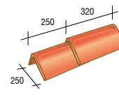
334 EM Shed-vorstpan - 4 per lm - 2,4 kg
