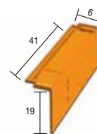
17 XLD Rechter gevelpan - 4,1 kg - 2,5 per lm
