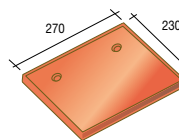
84 EL Ondervorstpan - 1,5 kg
