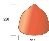
466 XL Kap zonder uitsnijding - 5,6 kg
