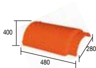
312 XG Cilindrische vorst 400 mm - 2,5 per lm - 4,8 kg
