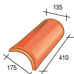
434 XLP Tapse noordboom (klein model) - 1,9 kg
