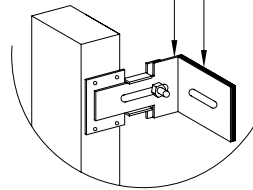
REGELBARE WINKELHAAK VENTISOL-LAT GALVA
