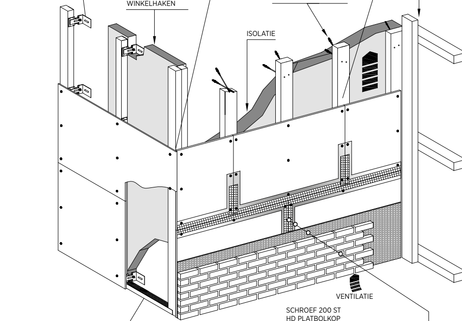
AFWERKING MET STEENSTRIPS - MEMBRAANPASTA OP VOEGEN - ALKALI-RESISTENTE VOEGBAND - LIJMMORTEL - STEENSTRIPS
