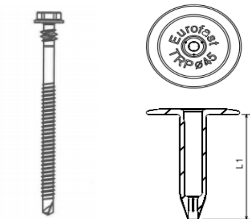
Fig. 6– Schroef VRF EUROFAST® EDS B + tule VRF EUROFAST® TRP45-L
