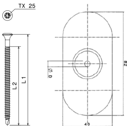
Fig. 4– Schroef VRF EUROFAST® EDS BZT + bevestigingsplaatje VRF EUROFAST® DVPEF8240D
