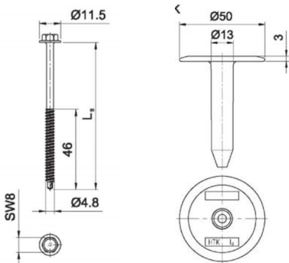
Fig. 7- Schroef EJOT DABO® TKR-4,8 + tule EJOT HTK
