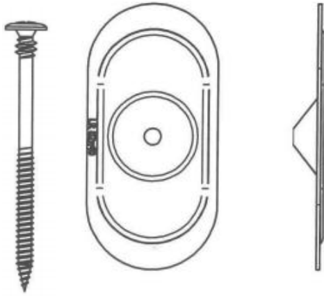
Fig. 3– Schroef LR ETANCO® EVDF 2C + bevestigingsplaatje LR ETANCO® 82x40 R DF
