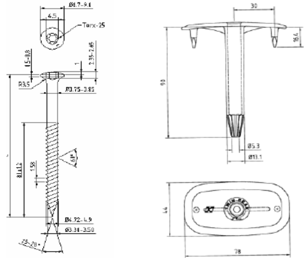
Fig. 5– Schroef SFS ISOTAK® PS-48 + tule SFS ISOFAST® TWIN PEAK PLUS
