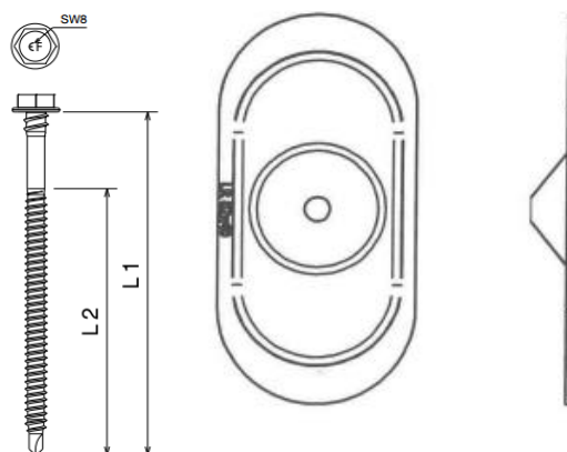
Fig. 2– Schroef LR ETANCO® EHB DF 2C + bevestigingsplaatje LR ETANCO® 82x40 R DF
