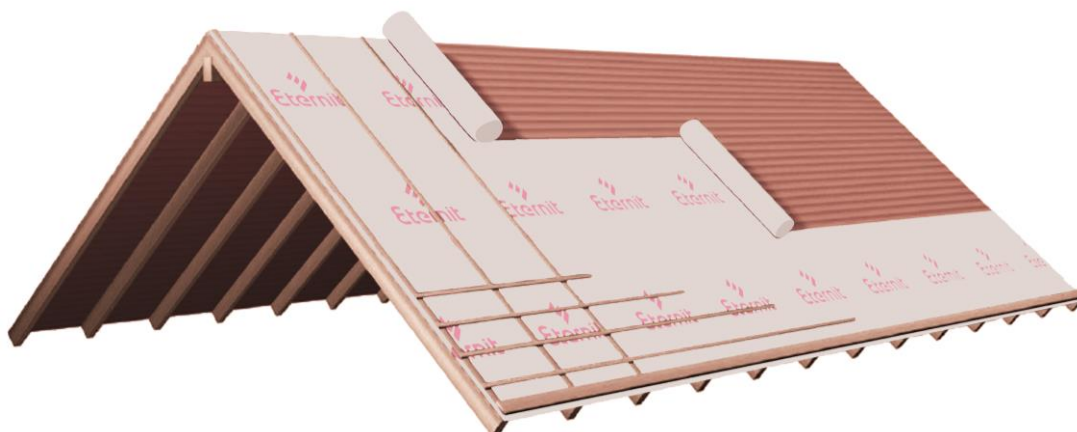
Fig. 2: DUO LONGLIFE EXTRA posé en contact direct d'un support en bois
