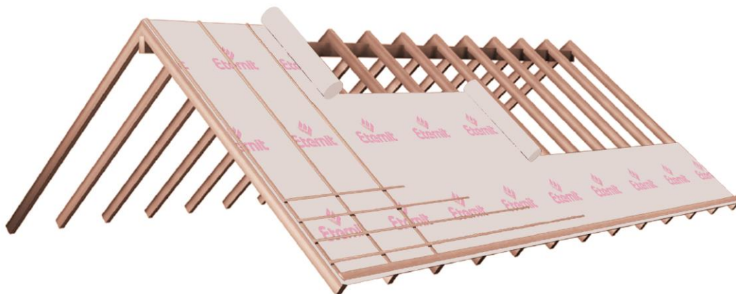
Fig. 1: DUO LONGLIFE EXTRA posé directement sur les chevrons
