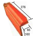
16 CFPV Linker gevelpan Côte Fleurie PV - 3,5 per lm - 2,1 kg
