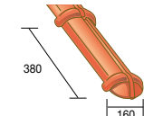
881 XL Stijlvolle eindnoordboom (klein model) - 2,2 kg
