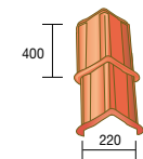
32 XL Brede noordboom met sluiting (groot model) - 2,6 per lm - 3,2 kg
