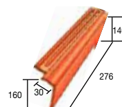
17 CFPV Rechter gevelpan Côte Fleurie PV - 3,5 per lm - 2,1 kg
