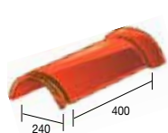
31 XL Halfronde ventilerende sluitvorst - 2,5 per lm - 4,1 kg
