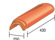
392 XL Halfronde ventilerende eindsluitvorst - 3,6 kg
