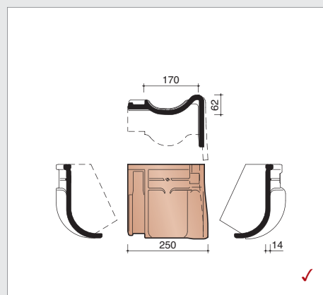
P4017290 Tuile membron de rive droite
