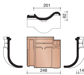
P4018200 5 pièces/m crt Tuile membron
