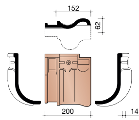
P4018230 Tuile membron trois quart
