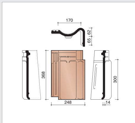
P4017090 3,4 pièces/m crt Tuile de rive droite
