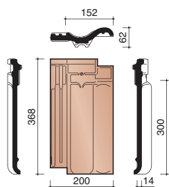
P4018030 3,4 pièces/m crt Tuile trois quart
