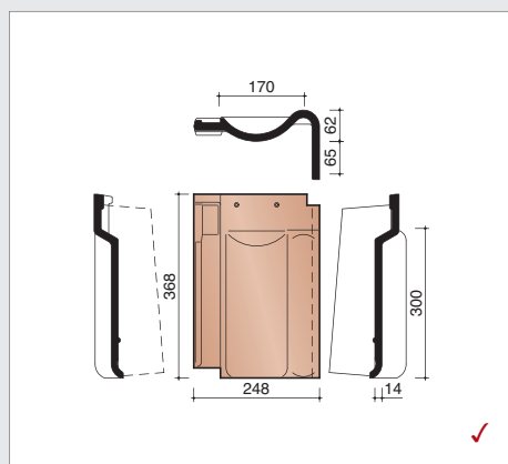
P4017190 Tuile de rive droite sous-faîtière
