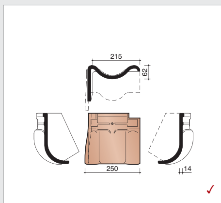
P4017280 Tuile membron de rive gauche
