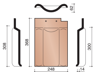
P4018150 Tuile sous-faîtière à double bourrelet
