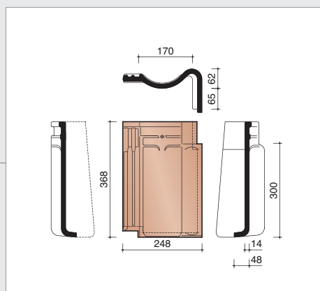
P4017390 Tuile de rive droite à bord recourbé
