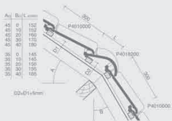
Plan de pose longitudinale de la toiture au niveau de la tuile membron
