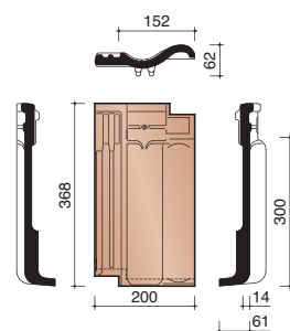
P4018330 Tuile trois quart à bord recourbé
