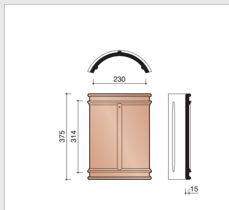
P0001230 Faîtière demi-ronde à double emboîtement - 230 mm
