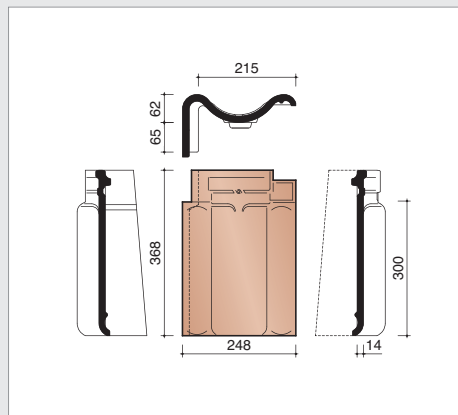
P4017080 3,4 pièces/m crt Tuile de rive gauche
