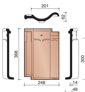
P4018300 5 pièces/m crt Tuile à bord recourbé
