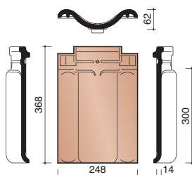
P4018050 3,4 pièces/m crt Tuile à double bourrelet
