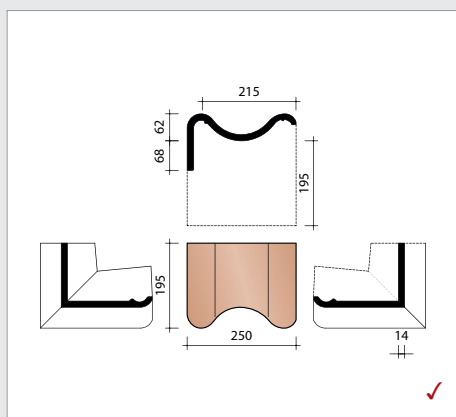
P4017580 Tuile faîtière de rive gauche (collée)
