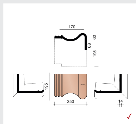
P4017590 Tuile faîtière de rive droite (collée)
