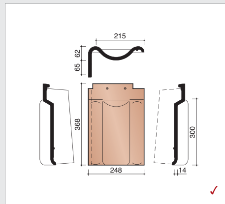
P4017180 Tuile de rive gauche sous-faîtière
