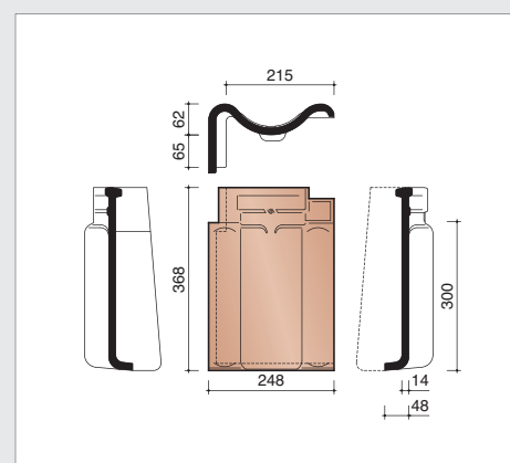
P4017380 Tuile de rive gauche à bord recourbé
