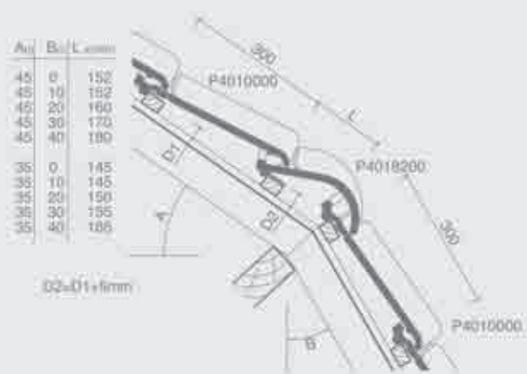
Lengtedoorsnede dak ter hoogte van knikpan
