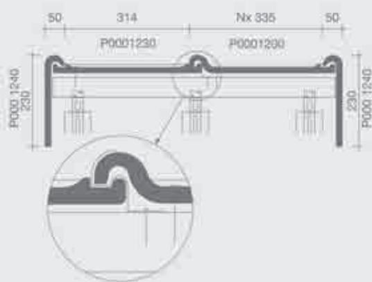
Dwarsdoorsnede dak ter hoogte van vorst 1200
