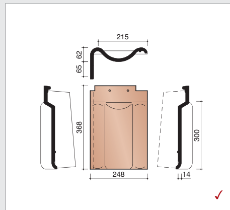
P4017180 Linker ondervorstgevelpan
