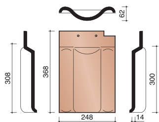
P4018150 Ondervorstpan met dubbele wel
