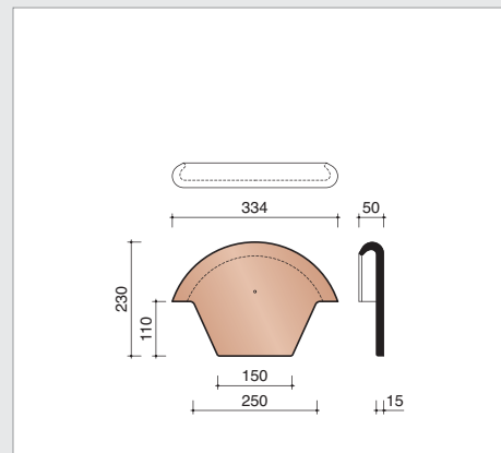
P0001240 Kopplaat - 230 mm
