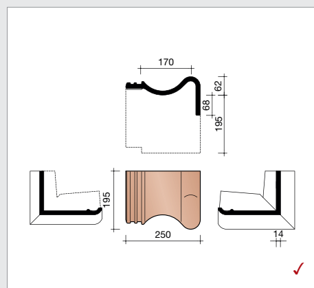
P4017590 Rechter gevelhaakvorst (verlijmd)
