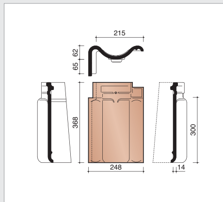
P4017080 3,4 stuks/lm Linker gevelpan
