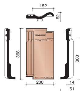
P4018330 Driekwart pan met gebogen boord
