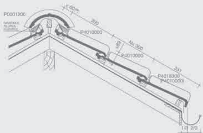
Lengtedoorsnede dak ter hoogte van vorst - met ondervorstpan
