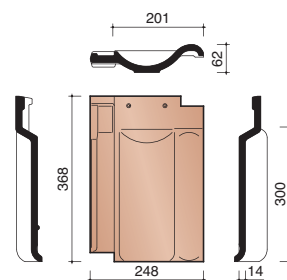
P4018100 5 stuks/lm Ondervorstpan
