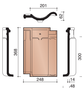
P4018300 5 stuks/lm Pan met gebogen boord
