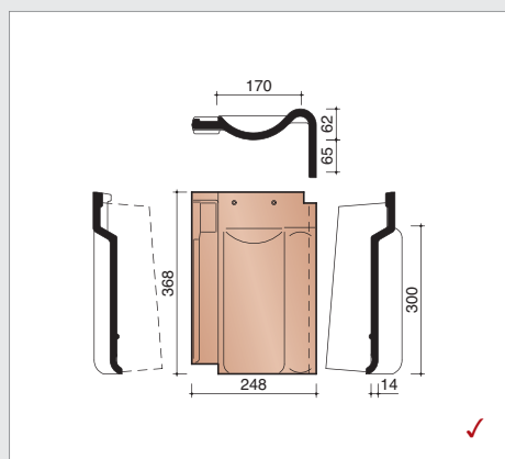
P4017190 Rechter ondervorstgevelpan
