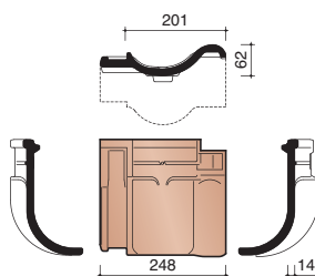
P4018200 5 stuks/lm Knikpan
