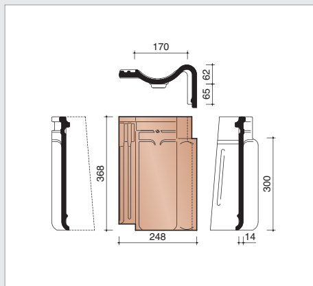
P4017090 3,4 stuks/lm Rechter gevelpan
