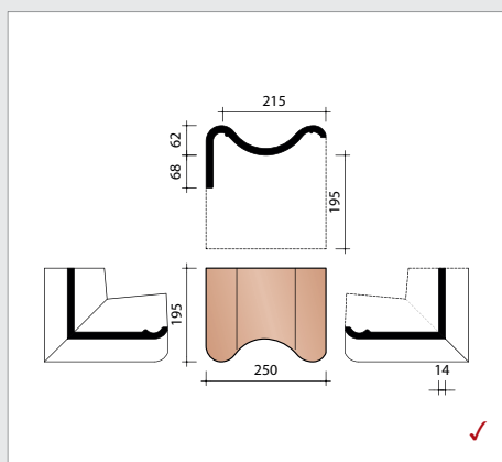
P4017580 Linker gevelhaakvorst (verlijmd)
