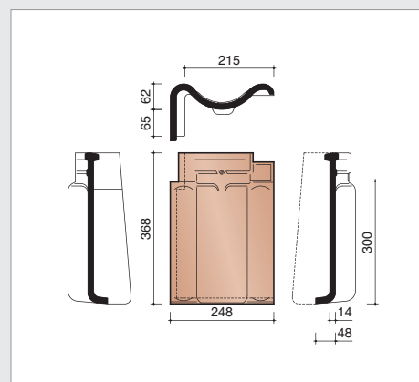
P4017380 Linker gevelpan met gebogen boord
