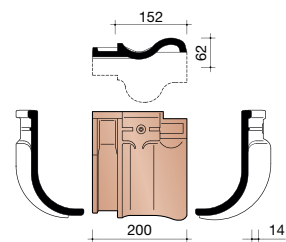
P4018230 Driekwart knikpan
