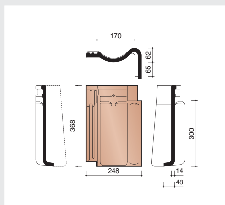
P4017390 Rechter gevelpan met gebogen boord
