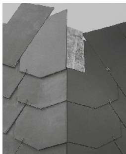
Arêtier avec ardoises taillées en biais
