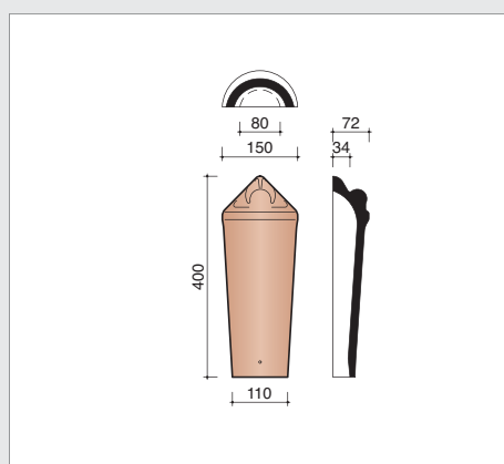
A0003810 About d'arêtier de chevauchement
