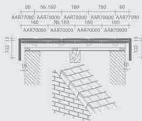
Plan de pose transversale de la toiture au niveau du pignon avec des tuiles posées au mortier
