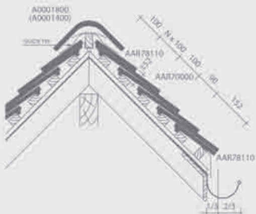
Plan de pose longitudinale de la toiture au niveau de la faîtière - Quick fix
