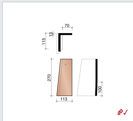
AAR77080 5 pièces/m crt Tuile de rive gauche
