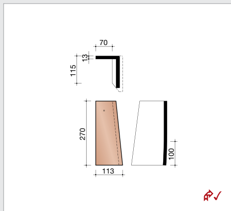
AAR77090 5 pièces/m crt Tuile de rive droite
