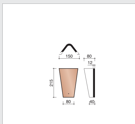
A0003700 10 pièces/m crt Cornier
