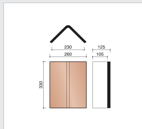
A0001800 3 pièces/m crt Faîtière angulaire
