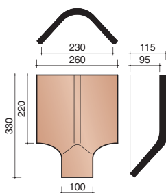
A0005800 Jonction entre 1 faîtière 1800 et 2 arêtiers 3700
