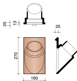
AAR78720 Tuile à douille Ø 100 mm
