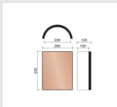
A0001400 3 pièces/m crt Faîtière demi-ronde
