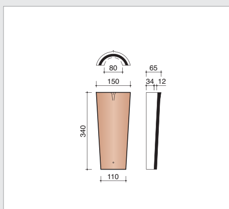
A0003800 3,5 pièces/m crt Arêtier de chevauchement
