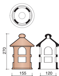
AAR78730 Mitron pour tuile à douille Ø 100 mm
