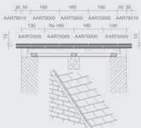
Plan de pose transversale de la toiture au niveau du pignon avec des tuiles posées au mortier
