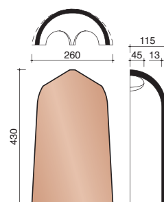
A0005880 Jonction entre 1 faîtière 1400 et 2 arêtiers 3700 / 3800
