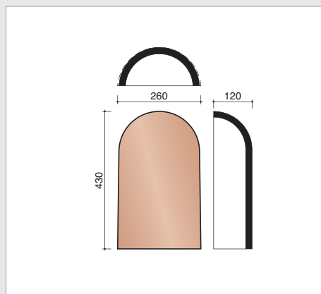
A0001420 About de faîtière demi-ronde - début et fin
