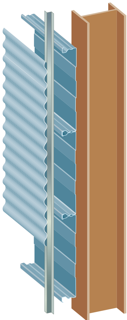
verticale montage
