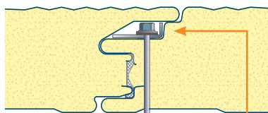
Verborgene bevestiging
