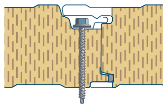
Verborgen bevestiging
